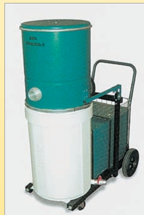
SPANGESOG Φορητή σκούπα για καθαρισμό εργαλειο- μηχανών, με δυνα- τότητα αναρρόφησης και διαχωρισμού των υγρών ψύξης τα οποία μπορούν να ξαναχρη- σιμοποιηθούν
