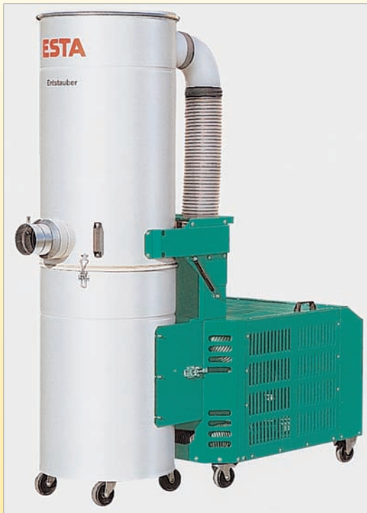
DUSTOVAC Φορητή σκούπα υψηλού κενού δυναμικότητας από 480-1100 m 3 /h με στατική πίεση μέχρι 25.000 pa
